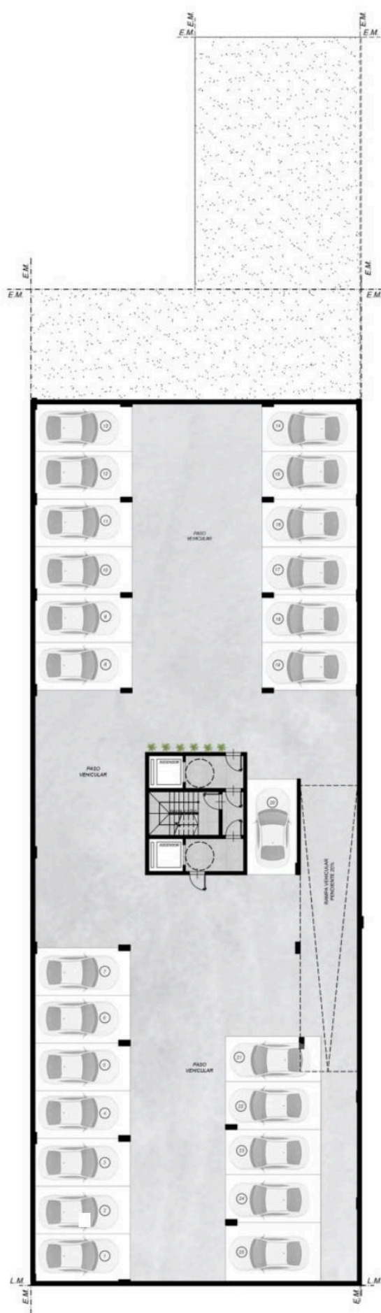
PLANTA SUBSUELO
